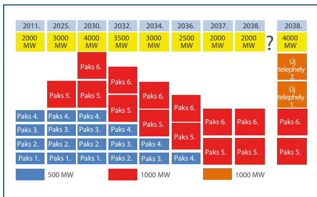
13. ábra: Magyarország nukleáris kapacitásainak várható alakulása 2038-ig (NFM 2012)
